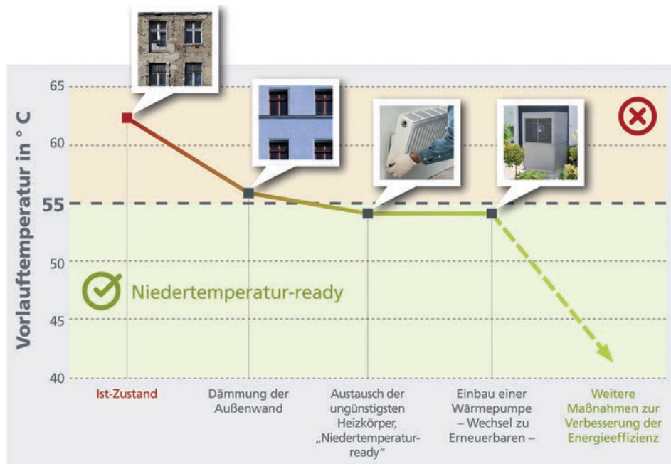
Ein Bündel von Maßnahmen ermöglicht den Einsatz von regenerativen Energien im Gebäudebestand. Quelle: VDPM
