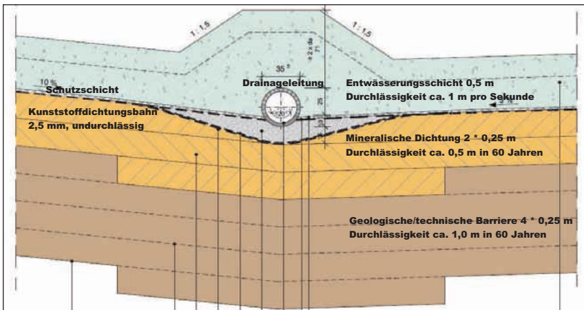
Aufbau der Basisabdichtung der Deponie
